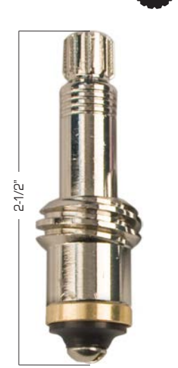
18 FISHER® 54518 • 54526 Hot w/handle (OEM) ▲680728 Cold w/handle (OEM) ▲680729
